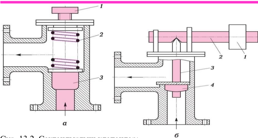
Сур. 13.2. Сақтандырғыш клапандар:
