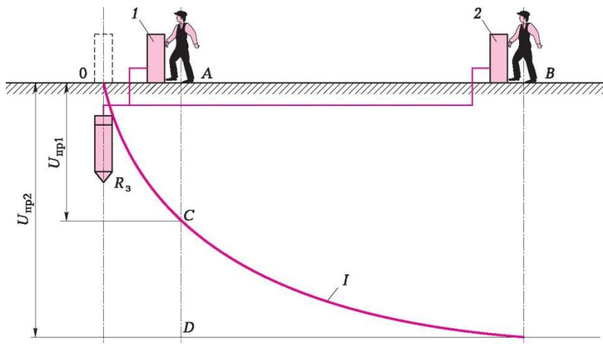
Сур 17.6 Кернеуге жанасу 1,2 электроқондырғылар
