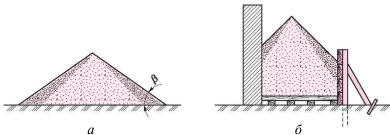
Сур. 7.8. Сырғымалы бос материалдарды сақтау:
