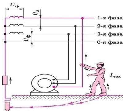
Сур. 17.1. Үшфазалы ток тізбегінде адамның бірфазаға қосылу схемасы: U — фазалық кернеу; U_{\text{п}} — желілік кернеу; I_{\text{адам}} — адам арқылы өтетін, ток күші
