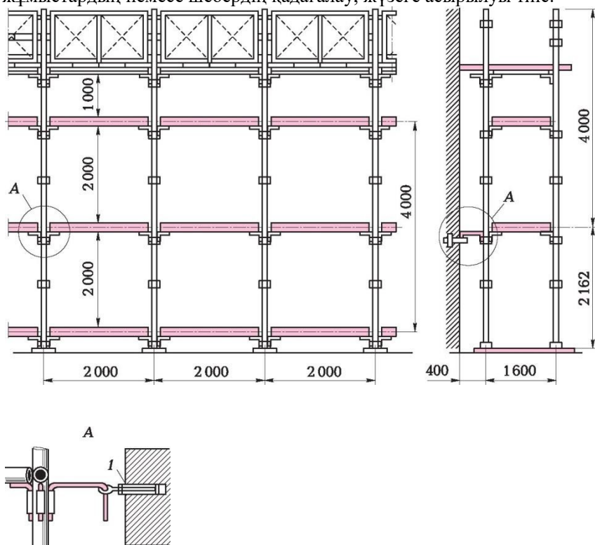
Сур. 15.2. Тұрбалы болтсыз лесалар:
