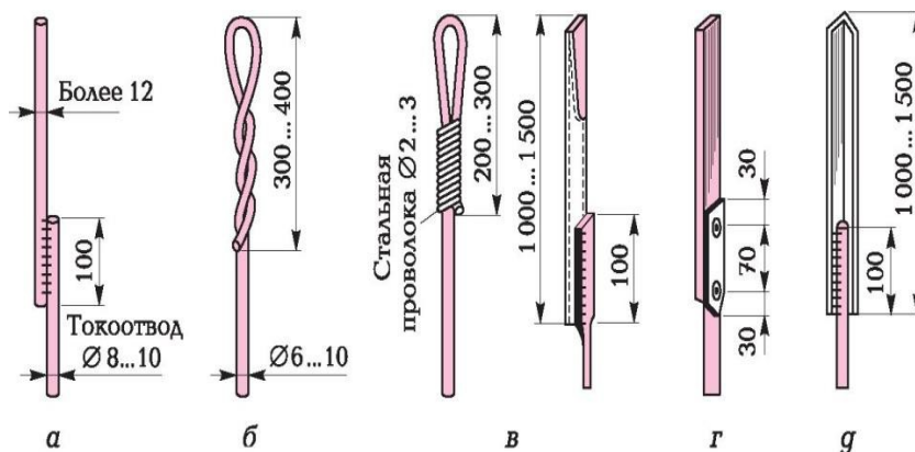
7.12 .сур. Найзағай қабылдау стержендерінің найзағай қағу конструкциясы: а — дөңгелек болат стержендерден; б — жіңішке болат сымдардан; в — болат тұрбалардан; г, д — түрлі болат профилдерден.
