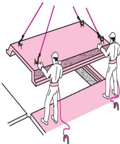
Сур 9.1. Жаппа жабудағы монтажниктердің қауіпсіз жерге тұруы
