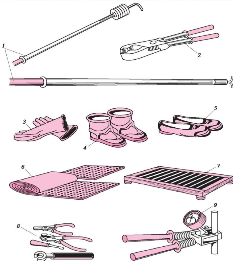
Сур.17.10. Электроконтрығыларда қолданылатын қорғану құралдары:
