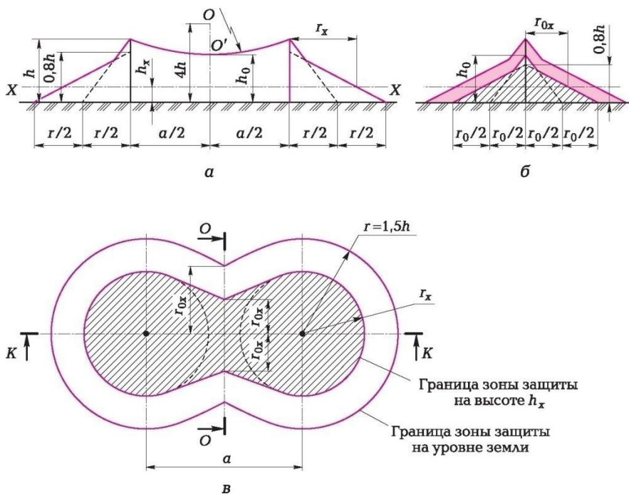
Сур 7.14. Антена найзағайының қорғау аймағының тік (а), көлденең (б) және қиғаш (в) аумақтары
