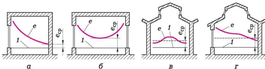
Сур. 18.5. а — бір жақты жанама жарық; б — екі жақты жанама жарық; в — жоғарғы жарық; г — аралас жарық; 1 — жұмыс жазықтығының деңгейі; e_{\min} және e_{\text{ср}} — табиғи жарық коэффициентінің төмен және орта мәнінің сәйкес келуі
