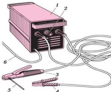
Сур 10.1. Электрлік дәнекерлеу жабдықтары:
