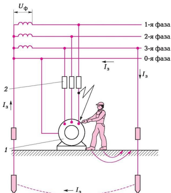
Сур. 17.7. Қорғаныш нөлдендіру іс-әрекетінің қағидатты схемасы: 1 — электродвигатель; 2 — сақтандырғыш
