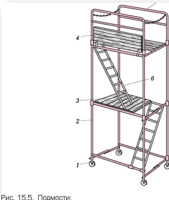
Рис. 15.5. Подмости:
